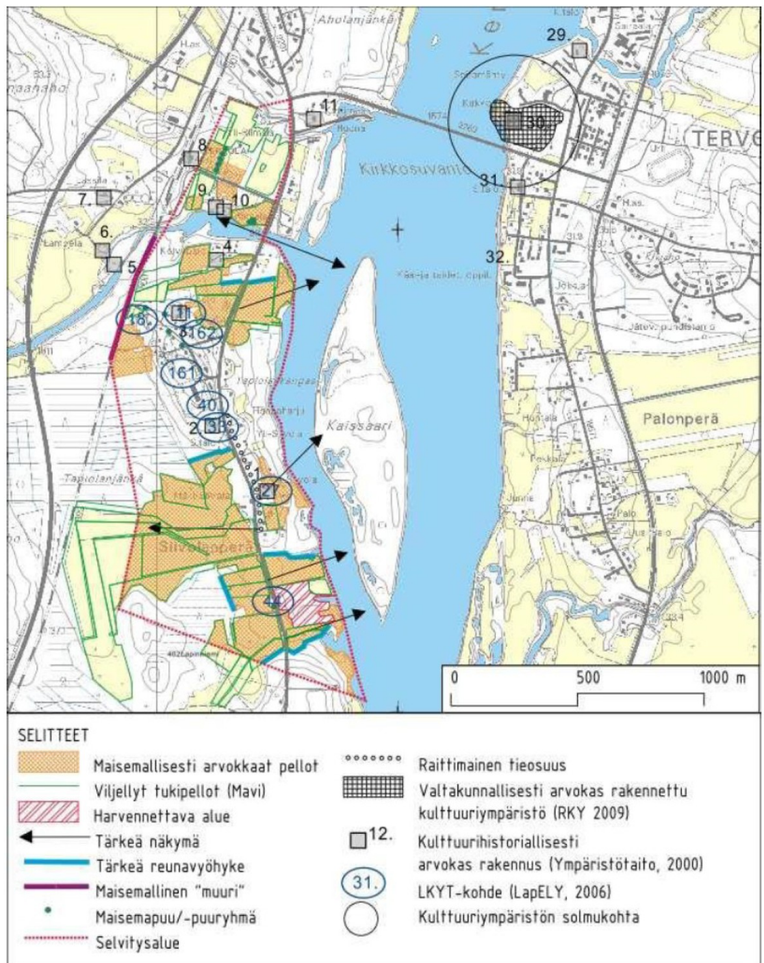
Kuva 9. Maisema-analyysi, Kaisajoki
