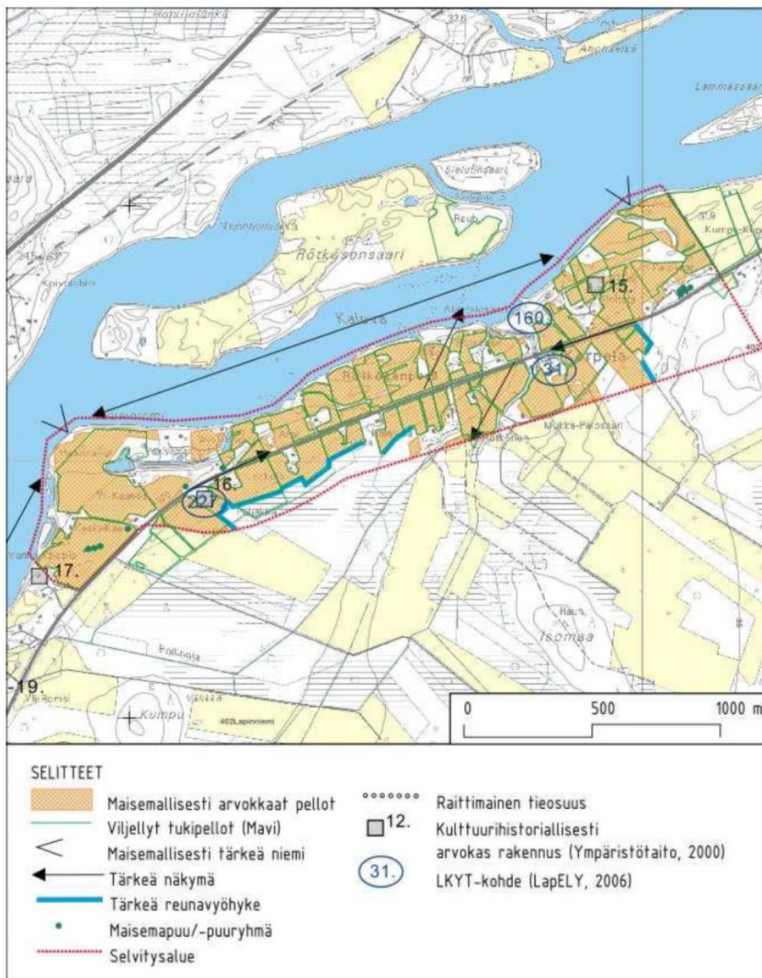
Kuva 10. Maisema-analyysi, Korpela.
