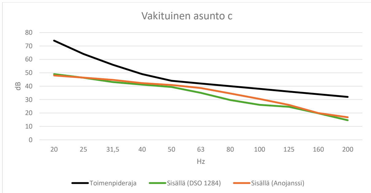
Kuva 5. Ympäristöministeriön ohjeistuksen mukainen pienitaajuisen melun laskenta sekä sosiaali- ja terveysministeriön toimenpiderajat vakituksessa asunnossa c.
