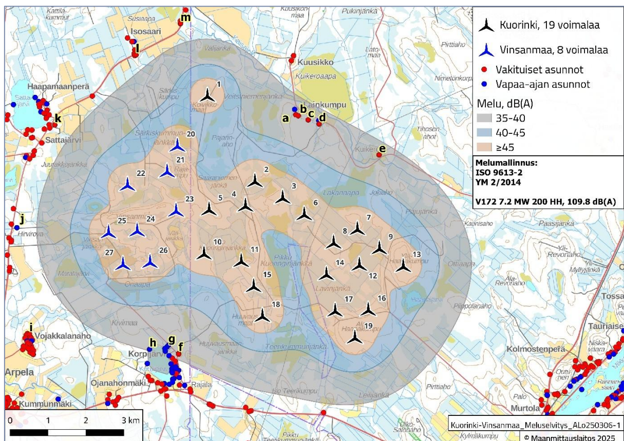
Kuva 1. Kuorinki-Vinsanmaan tuulivoimapaiston melumallinnus, V172 7,2 MW 200 m HH 109,8 dB(A). Kolmetaista havainnointipistettä on merkitty kuvaan kirjaimilla.
