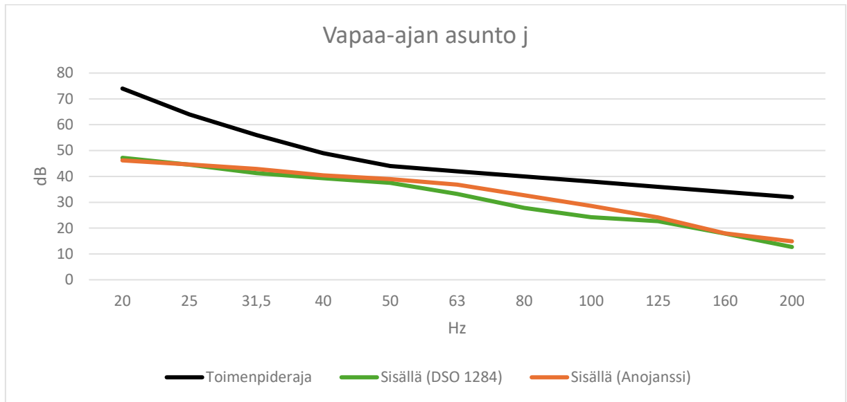
Kuva 6. Ympäristöministeriön ohjeistuksen mukainen pienitaajuisen melun laskenta sekä sosiaali- ja terveysministeriön toimenpiderajat vapaa-ajan asunnossa j.
