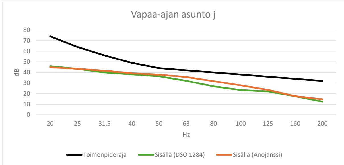
Kuva 4. Ympäristöministeriön ohjeistuksen mukainen pienitaajuisen melun laskenta sekä sosiaali- ja terveysministeriön toimenpiderajat vapaa-ajan asunnossa j.
