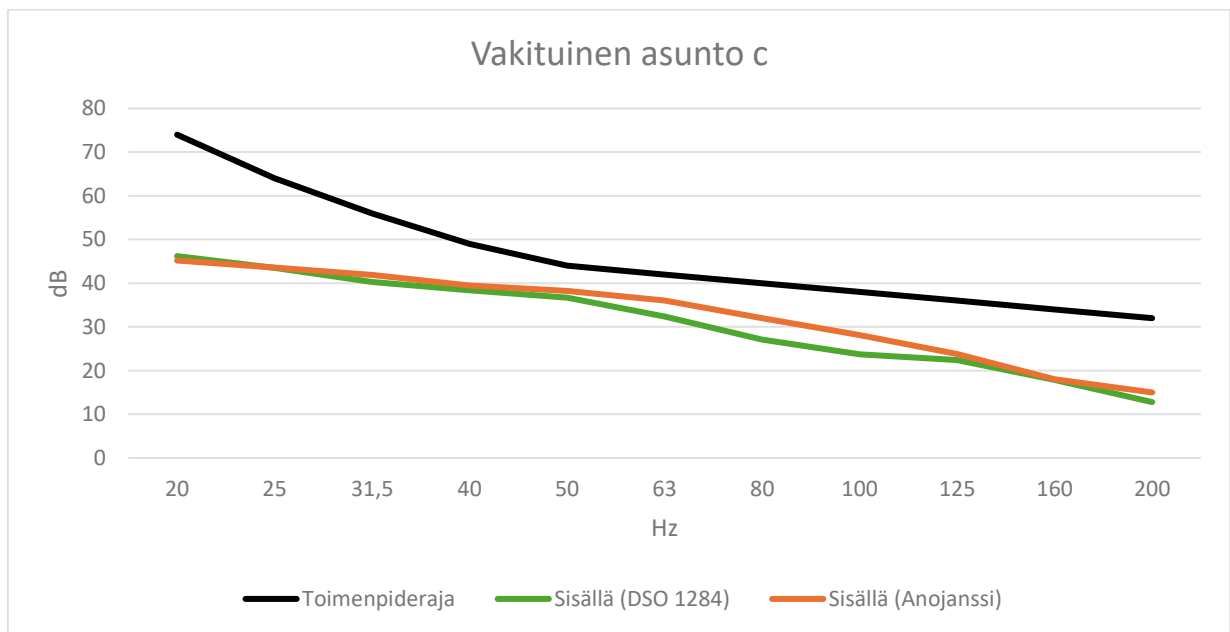
Kuva 3. Ympäristöministeriön ohjeistuksen mukainen pienitaajuisen melun laskenta sekä sosiaali- ja terveysministeriön toimenpiderajat vakituiseissa asunnossa c.
