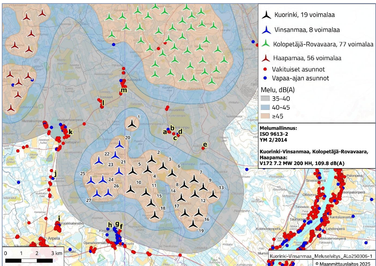
Kuva 2. Kuorinki-Vinsanmaan tuulivoimapuiston melumallinnus, V172 7,2 MW 200 m HH 109,8 dB(A). Kolmetoista havainnointipistettä on merkitty kuvaan kirjaimilla.
